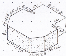
DETAĻU AKSONOMETRISKA SHĒMA:
