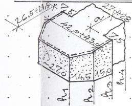
DETAĻU AKSONOMETRISKA SHEMA
