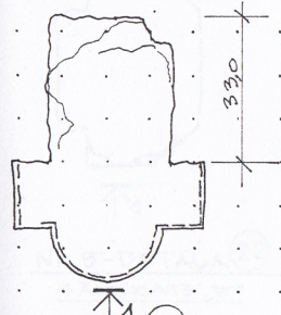
Nr.6-DETAĻA (30)
