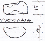
Nr.8-DETAĻA (102) PRETSKATS
