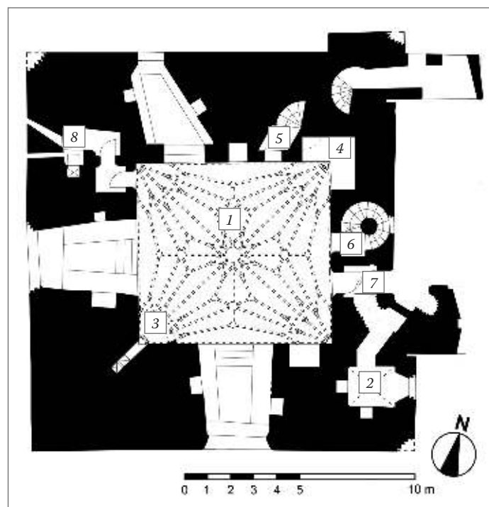
6. att. “Mestra istabas” plāns 1 – galvenā telpa; 2 – stūra telpa; 3 – kamīns; 4 – stūra niša; 5 – kāpnes uz leju; 6 – kāpnes uz augšu; 7 – eja uz dienvidu remteri; 8 – ateja K. Hermaņa zīmējums, 2021
